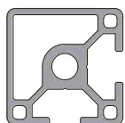
PROFILO SEZIONE 30x30 - 2 CAVE - 90°
