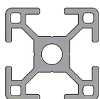
PROFILO SEZIONE 30x30 - 4 CAVE
