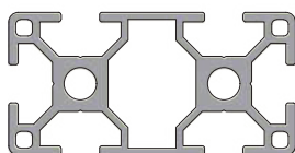
PROFILO SEZIONE 30x60 - 6 CAVE
