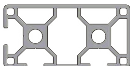
PROFILO SEZIONE 30x60 - 3 CAVE
