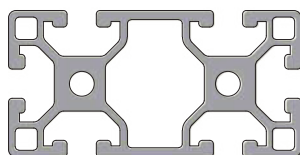
PROFILO SEZIONE 40x80 - 6 CAVE
