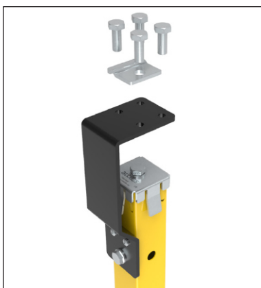
07 PLACA PARA FIJACIÓN EN REJILLA
