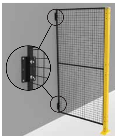
08 KIT COLLEGAMENTO PANNELLO-PARETE
